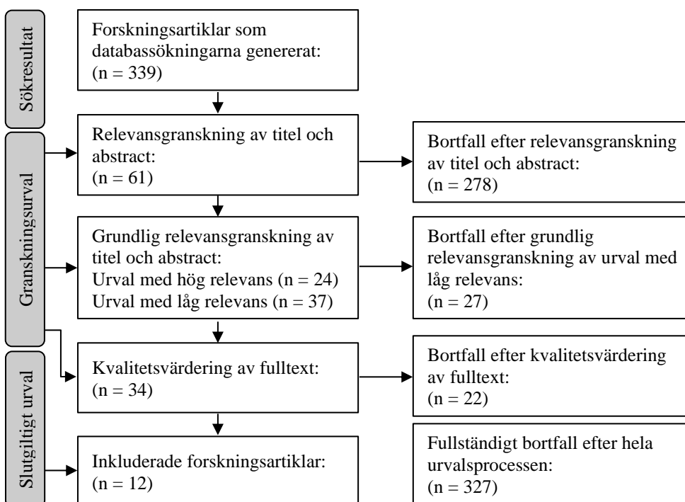
Figur 1: Flödesschema inspirerad av PRISMA Flow Diagram (PRISMA, 2021)
