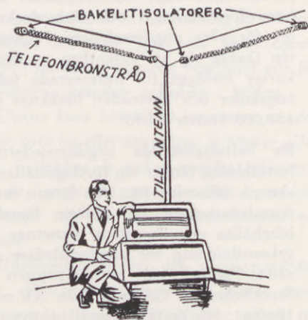
TFAE:s inomhusantenn
