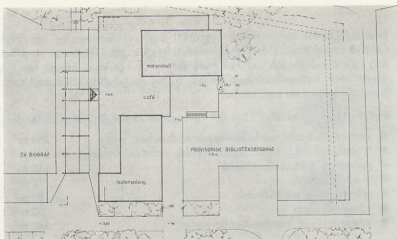
Situationsplan av fritidsgården
