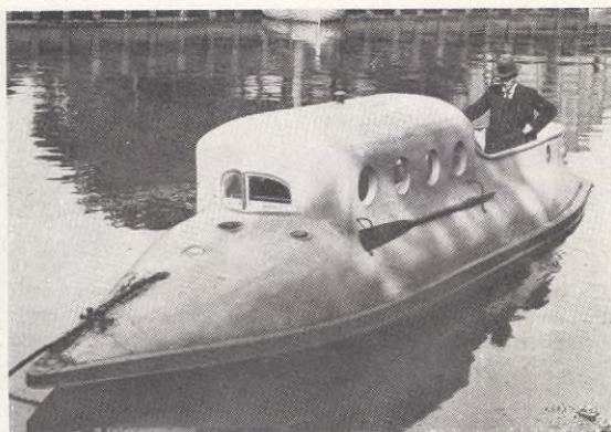
Central Ateliern, Malmö. Nichte: Ernst Sjöversparre. MOTORBÅT AF BETONG. SJÖSATT I MALMÖ.
