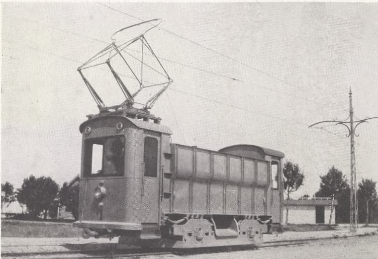
ELEKTRISK MOTORVAGN FÖR TRANSPORT AF KOL, KOKS, LERA o. d. Å Malmö SPÅRVÄGAR. Vagnen, den första i sitt slag, är byggd på Malmö Spårvägars verkstäder, lastar 8 ton och drager 2 släpvagnar för samma ändamål.
