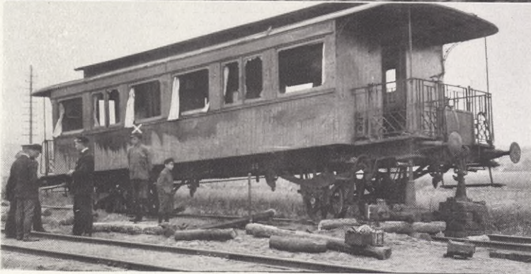
1. OLYCKSPLETSEN VID JÄRNBROTTS STATION MED TÅGSÄTTET OCH DEN KULLVRÄKTA SISTA VAGNEN, omedelbart efter olyckan. — (Efter fotograf.)
