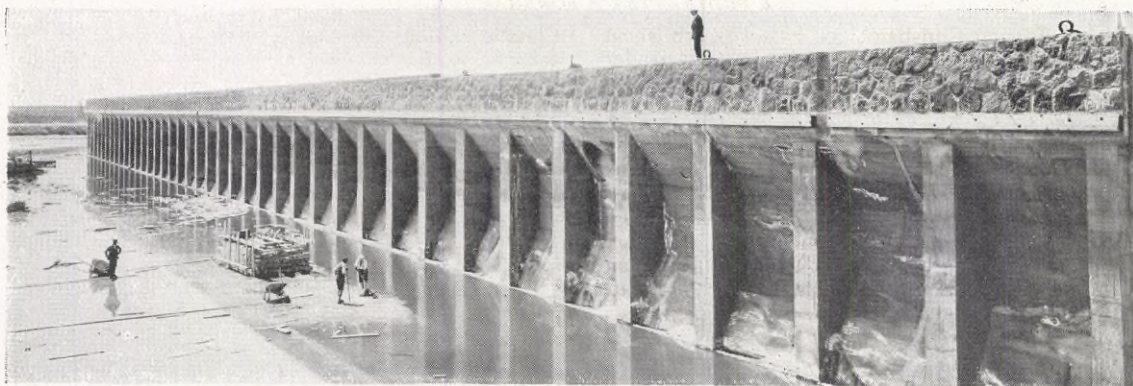
TEGELBRUKSHAMNEN UNDER TORRLÄGGNING. Kajmur och bålverk till bassängerna.
