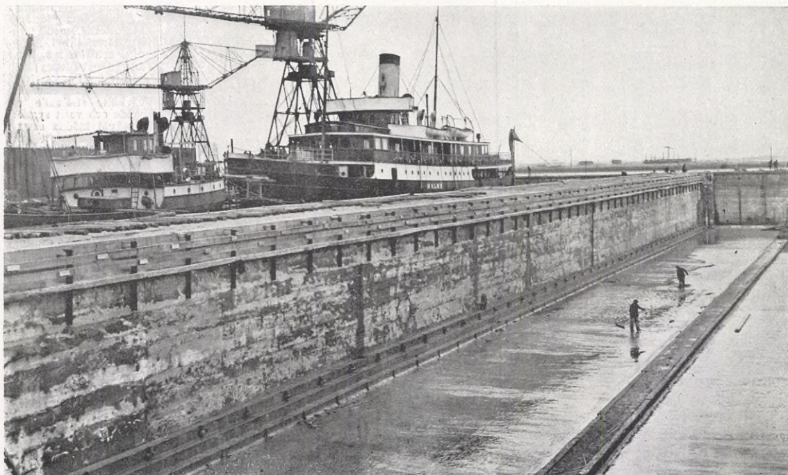
SYDHAMNEN. DEN SISTA AV DE STORA NYA DOCKORNA SOM NU ÄRO FÄRDIGA TAGAS I BRUK. I bakgrunden synes ångfärjan "Malmö" under reparation å det intill hamnanläggningen gränsande Baltica varvet.
