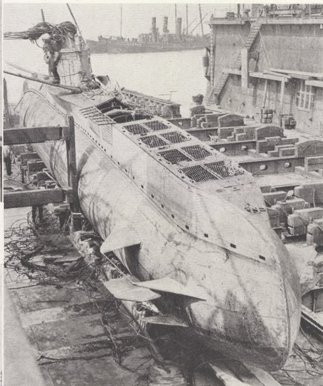
”U C. 5”, en tysk undervattens-minutläggare tagen och förd till England där den väckt stort uppspäende. Närmast synes de galleräckta förvaringsrummen för minorna.
