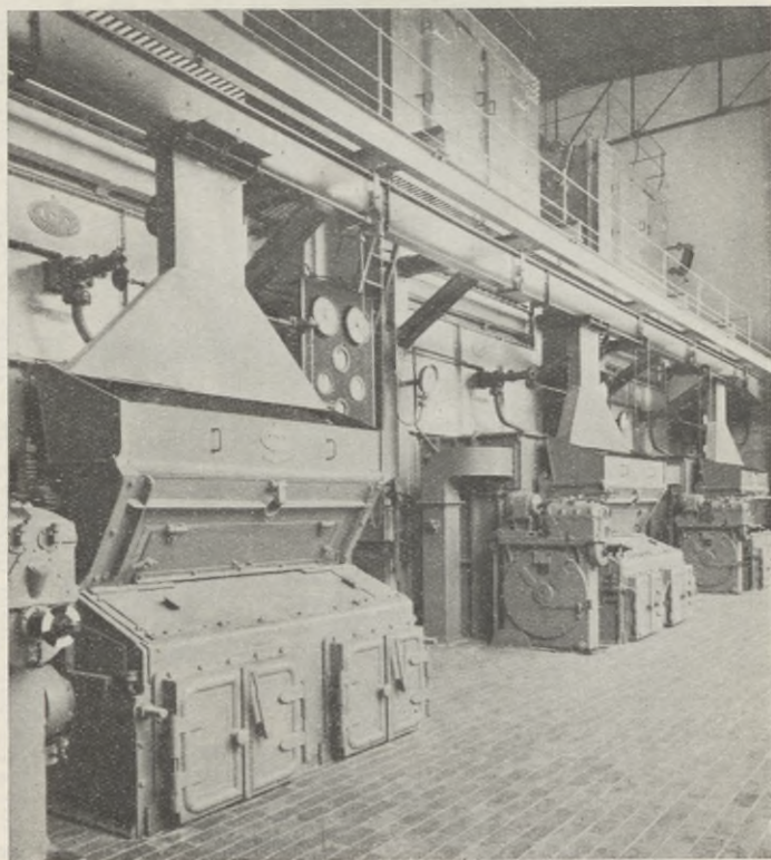
Ångpanneanläggningen.
