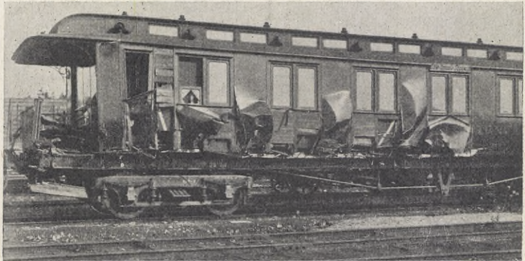
FRÅN TÅGURSPÅRINGEN VID GRANSTANDA Å GÄFLE-DALABANAN: Den ramponerade boggievagnen.
