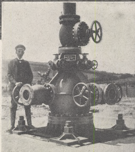
Efter fotografi. HUVUDGASKÄLLAN I KISSARMAS, afspärrad genom en ventil.
