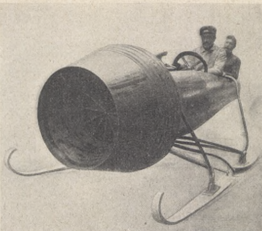
SLÄDAUTOMOBIL, UTFÖRD EFTER RITNINGAR AF STORFURST CYRILL AF RYSSLAND. Den beräknas kunna uppnå en hastighet af 100 km. i timmen på snö. Principen för dess framdrivande är hämtad från propellerens inverkan på ett aeroplan och realiserad på så sätt att en snabbgående turbinskiffva, hvilken under sin rotation lämnar den behöfliga dragkraften, monterats framtill.
