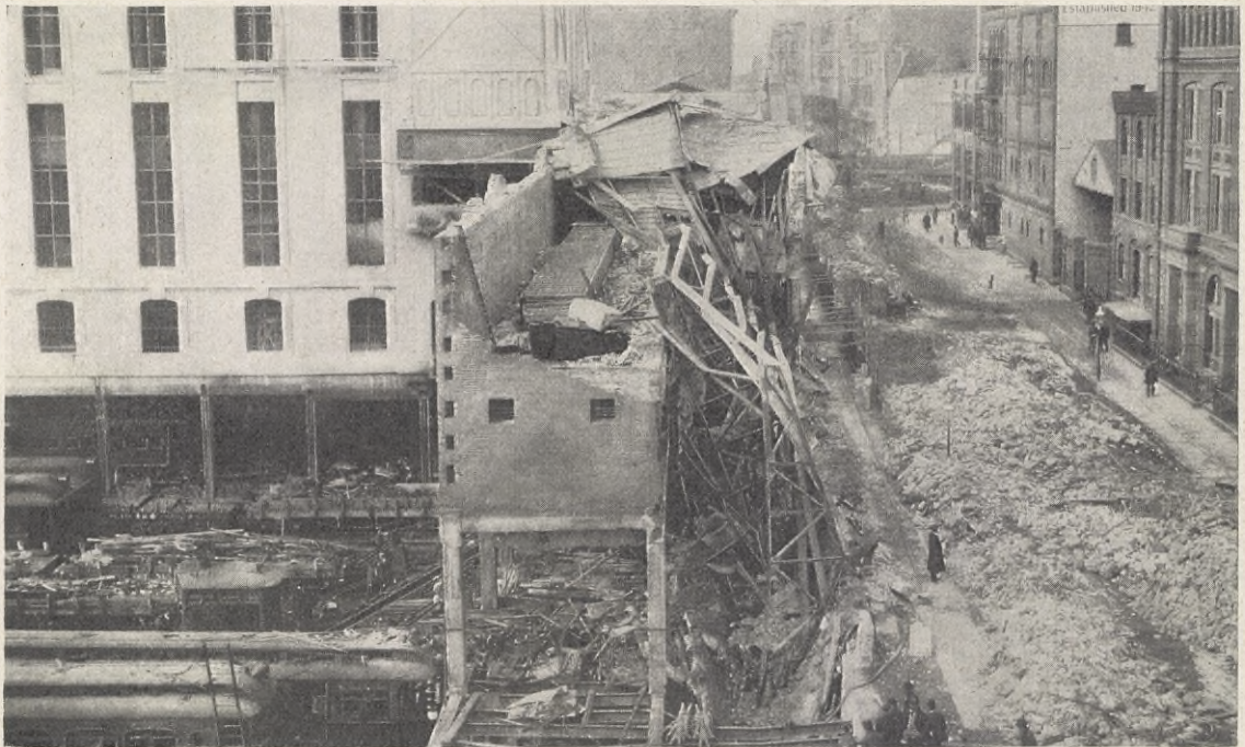
CENTRALBANANS KRAFTSTATION I NEW-YORK EFTER EXPLOSIONEN.
