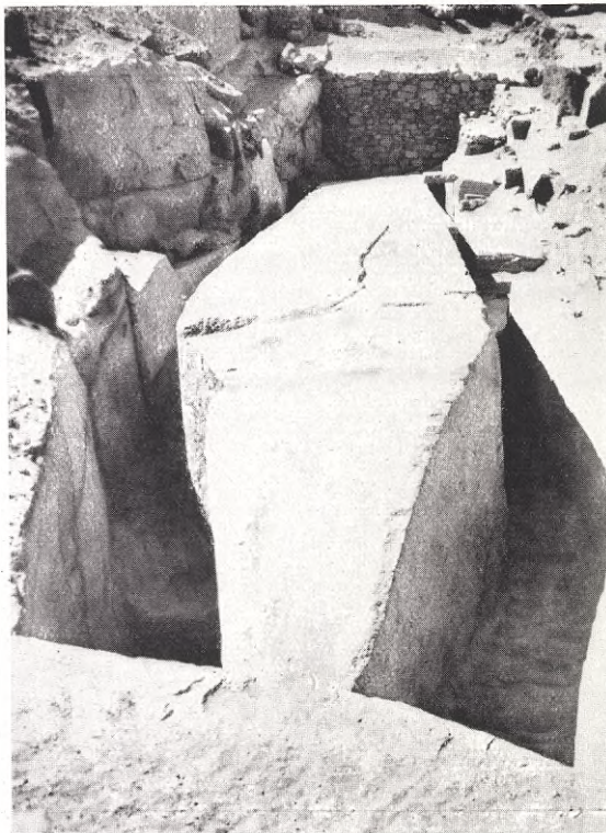
DEN STÖRSTA OBELISK SOM HITTILLS VARIT SEDD, NYUTGRÄVD I ASSUAN av Egyptiska fornminnesdepartementet. Denna jätteobelisk, ännu med spetsen fast vid det granitberg ur vilket den på sin tid blev uthuggen, mäter 40 meter i längd, 4,3 meter vid foten och 2,5 meter vid spetsen samt väger 1200 ton; motsvarande längd för Cleopatras nål, obeliskens i London, är 21 meter. — Efter fotografi. Kliché: Sjöberg, Gbg.
