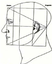
Figur 2. De Divina Proportione (Gyllene Snittet). (Pacioli, 1509).
