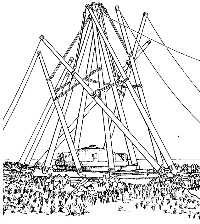
HYPOTETISK GRUNDKONSTRUKTION FÖR ATT KUNNA LYFTA MAUSOLEETS TAK. (KORRES 1997, s 252)
