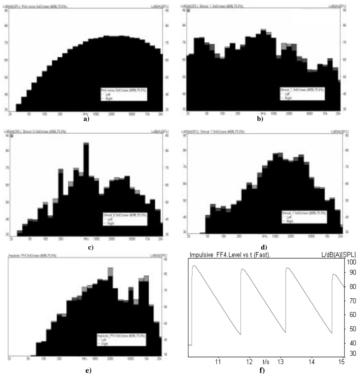
Figur 2.6. A-vägd tersbands spektrum för test signalerna (30 – 90 dB). a) Rosa brus. b) Lågfrekvent buller. c) Kompressorbuller med tonkontakt. d) Dieselmotorbuller. e) Impulsivt buller och f) tidsignalen för impulsivt ljud om integrationstid “fast” används.
