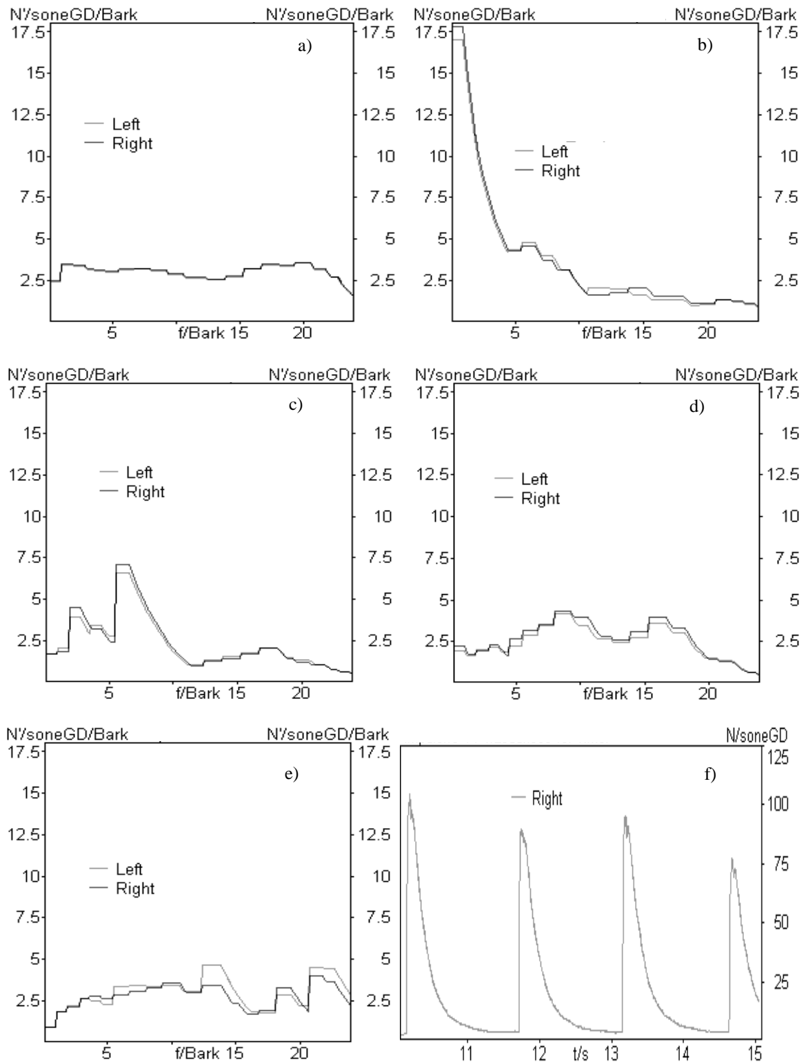
Figur 2.7. Specifik hörstyrka för de fem testsignalerna. Arealen under kurvan motsvarar total hörstyrka. En fördubbling av arean motsvarar en fördubbling av hörstyrkan. a) Rosa brus. b) Lågfrequent buller. c) Kompressorbuller med tonkaraktär. d) Dieselmotorbuller. e) Impulsivt buller och f) hörstyrkans variation över tiden för impuls ljudet.
