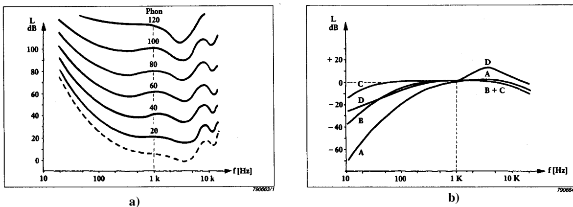
Figur 2.1. a) Lika-hörnivå-kurvor för sinustoner enligt ISO 226 (1966), b) standardiserade vägningskurvor, (Bruel & Kjaer 1986).
